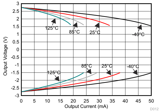
图 5-7. 输出电压与输出电流间的关系 ( 负载 )
