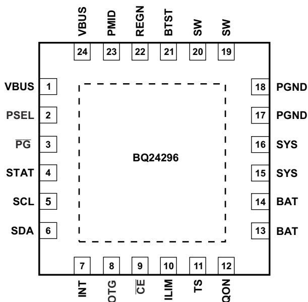
图 7-1. 24-Pin VQFN RGE Package (Top View)
