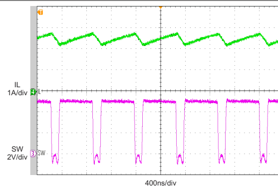
图 10-6. Charge Enable
