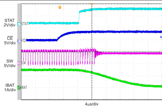
图 10-7. Charge Disable
