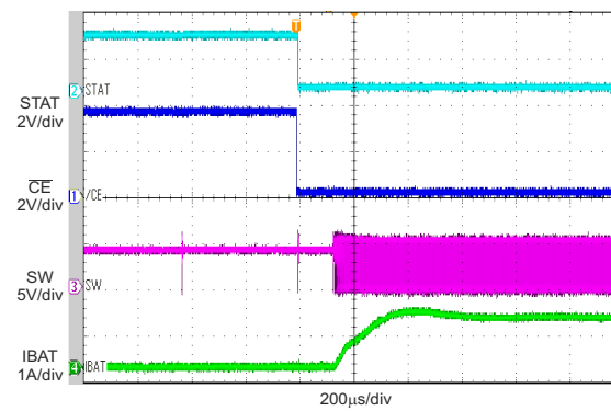
图 10-4. BQ24297 Power Up with Charge Enabled
