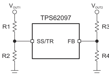
图 8-2. Output Voltage Tracking
