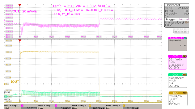
图 8-22. Load Transient, 100 mA Step
