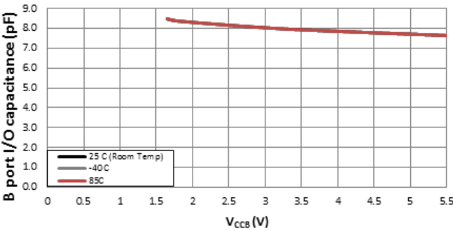
图 5-3. B 端口 I/O 引脚的电容 (C IO ) 与电源 (V_CCB)
