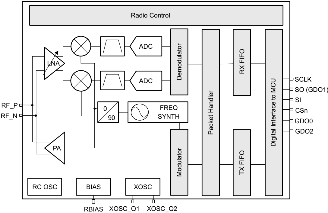
图 1-1. 功能框图
