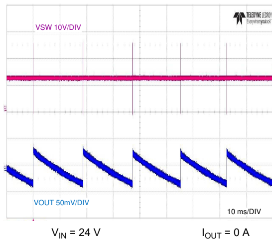
图 7-14. No-Load Switching
