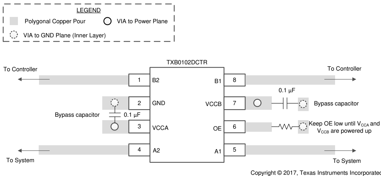
图 8-3. TXB0102 布局示例
