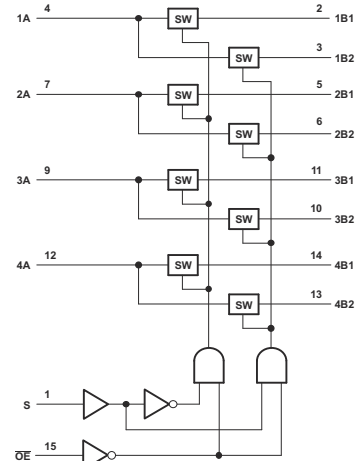
逻辑图 (正逻辑)
