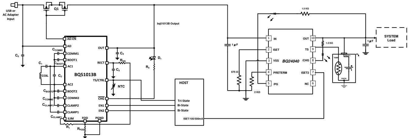
图 9-11. BQ51013B 用作无线电源供应适配器多路复用器，为线性充电器
