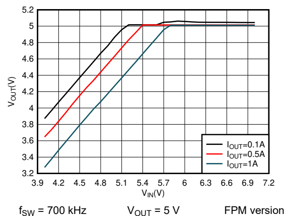
图 7-6. 5-V Dropout
