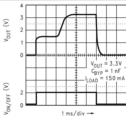
图 7-24. Turn-On Time (Legacy Chip)
