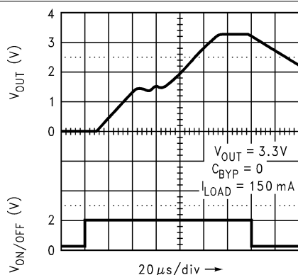
图 7-22. Turn-On Time (Legacy Chip)
