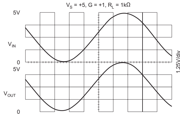
图 25. 轨至轨输入和输出
