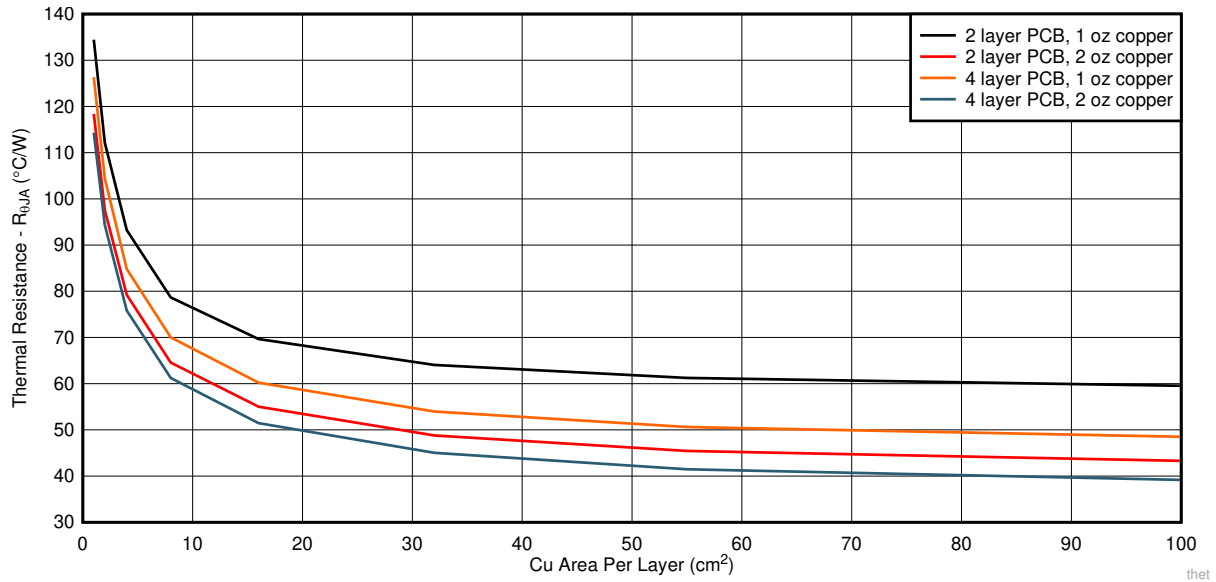
图 7-5. R_{\theta JA} 与铜面积的关系（DRV 封装）
