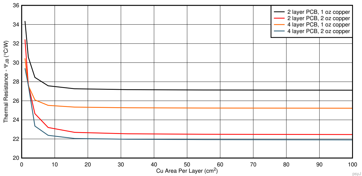
图 7-6. \psi_{JB} 与铜面积的关系（DRV 封装）
