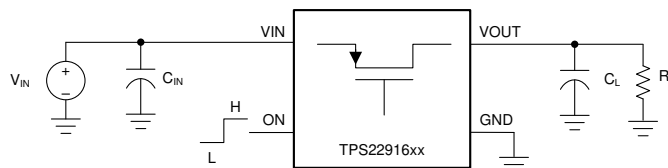
简化版原理图
