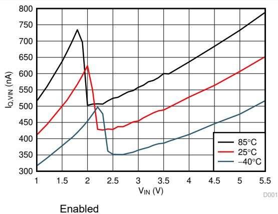
图 6-5. Quiescent Current
