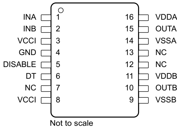
图 4-1. DW 封装 16 引脚 SOIC 顶视图
