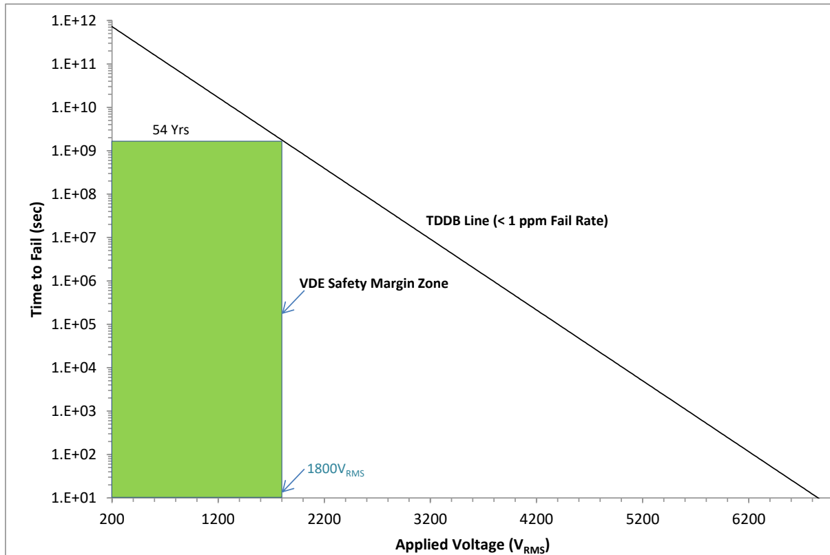
图 5-1. 增强型隔离电容器寿命预测
