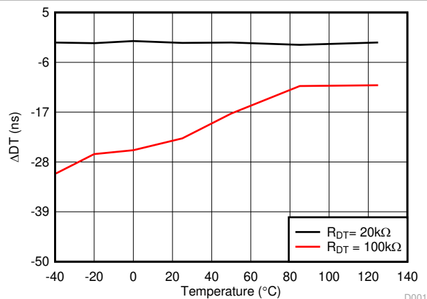
图 5-25. 死区时间匹配与温度之间的关系 ( R_{DT} = 20k\Omega 和 100k\Omega )
