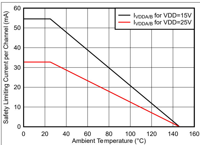
图 5-2. 安全相关限制电流的热降额曲线 (两个通道同时运行时每个通道的电流)
