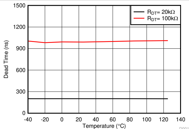
图 5-24. 死区时间与温度之间的关系 ( R_{DT} = 20k\Omega 和 100k\Omega )
