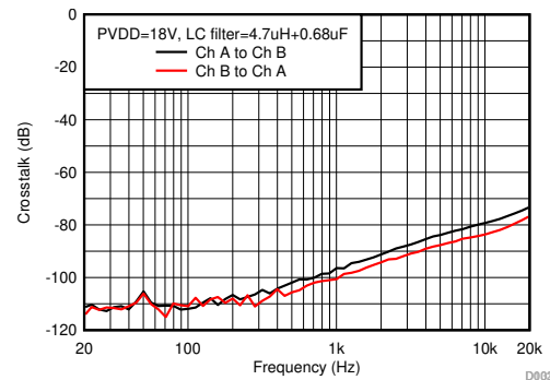
图 6-28. Crosstalk
