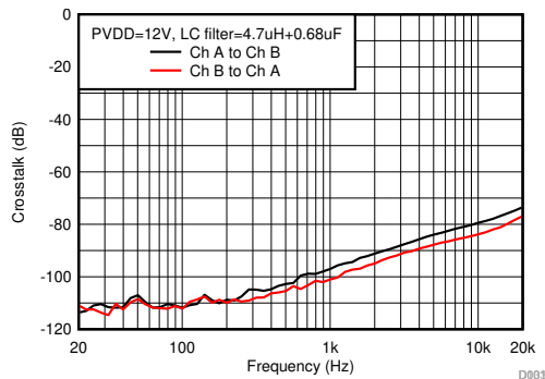
图 6-27. Crosstalk
