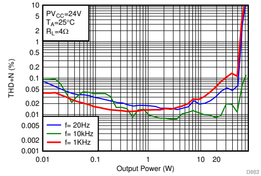
图 6-74. THD+N vs Output Power-PBTL
