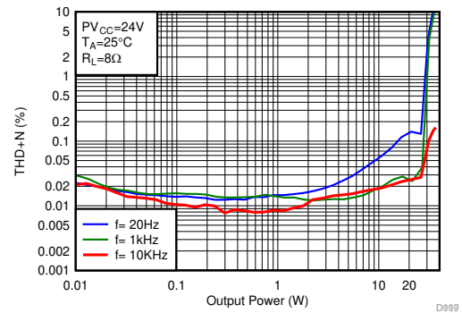
图 6-22. THD+N vs Output Power-BTL
