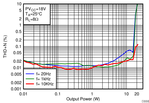
图 6-21. THD+N vs Output Power-BTL
