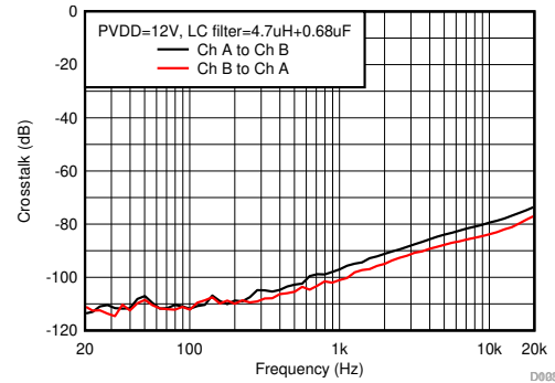
图 6-26. Crosstalk
