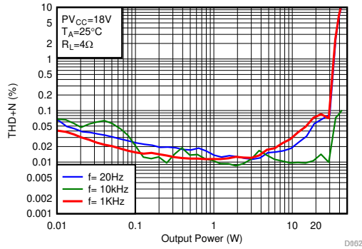
图 6-73. THD+N vs Output Power-PBTL
