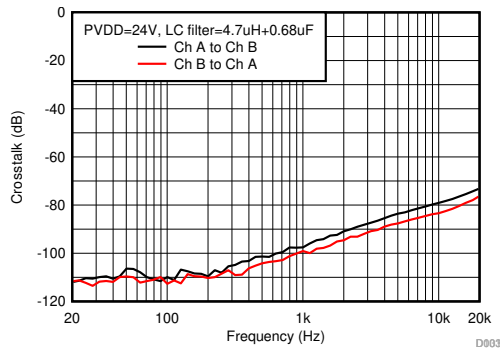
图 6-31. Crosstalk
