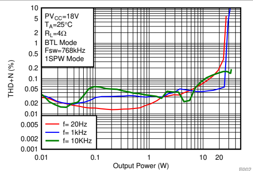
图 6-16. THD+N vs Output Power-BTL
