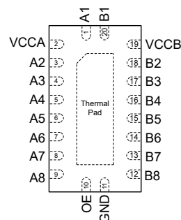
图 4-4. RKS 封装, 20 引脚 VQFN (顶视图)
