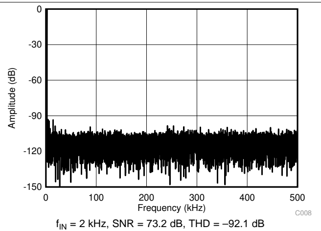
图 4. Typical FFT
