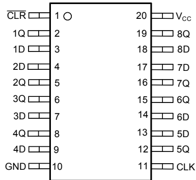
DB、DW、N、NS 或 PW 封装 20 引脚 SSOP、SOIC、PDIP、SO 或 TSSOP (顶视图)
