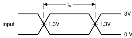
图 6-2. 电压波形，TTL 兼容型 CMOS 输入脉冲持续时间
