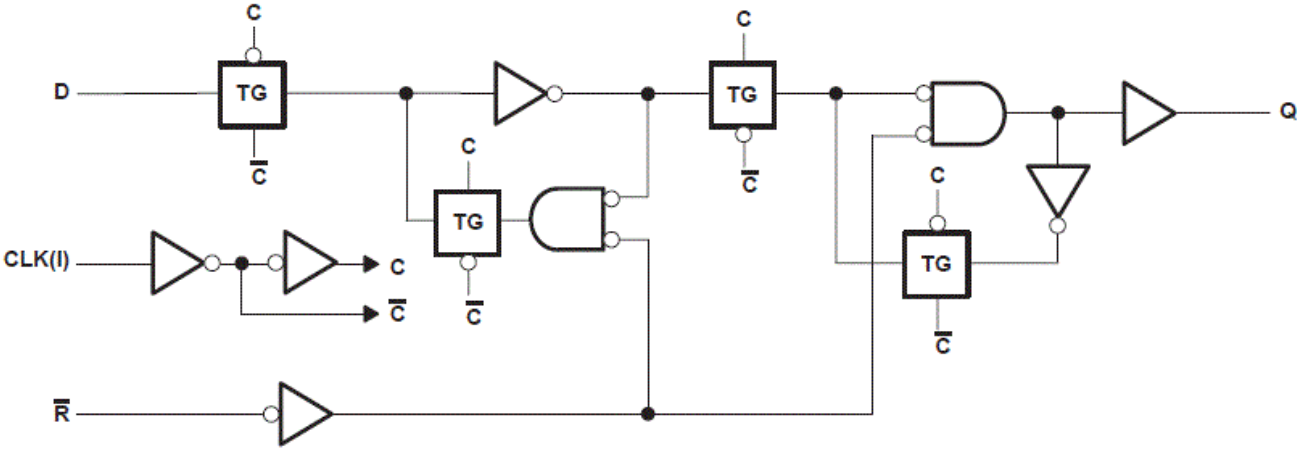
图 7-2. 展示各触发器的逻辑图 (正逻辑)
