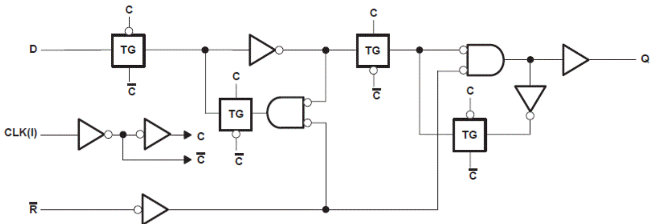
展示各触发器的逻辑图 (正逻辑)
