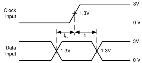
图 6-3. 电压波形，TTL 兼容型 CMOS 输入建立和保持时间
