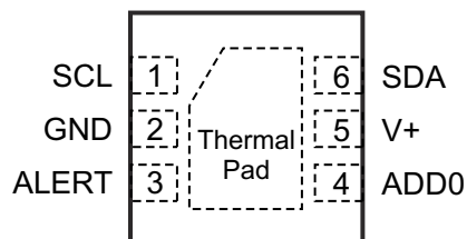
图 5-1. DRV 封装 6 引脚 WSON 顶视图
