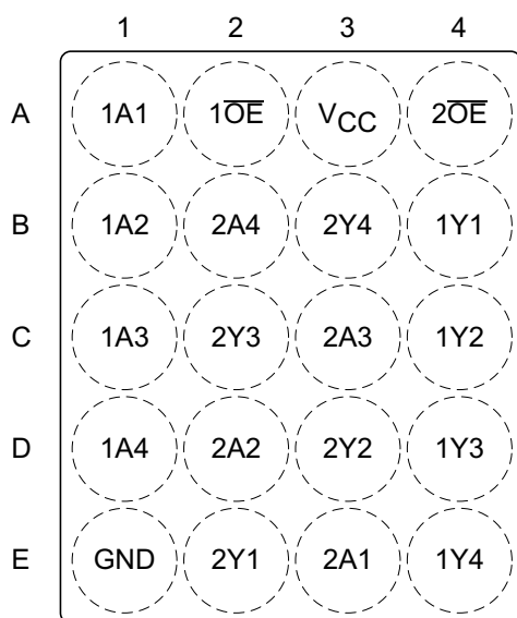
图 4-1. ZQN 封装 20 引脚 BGA 顶视图
