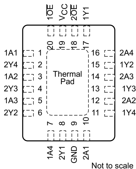
图 4-4. RWP 封装 20 引脚 X1QFN 顶视图
