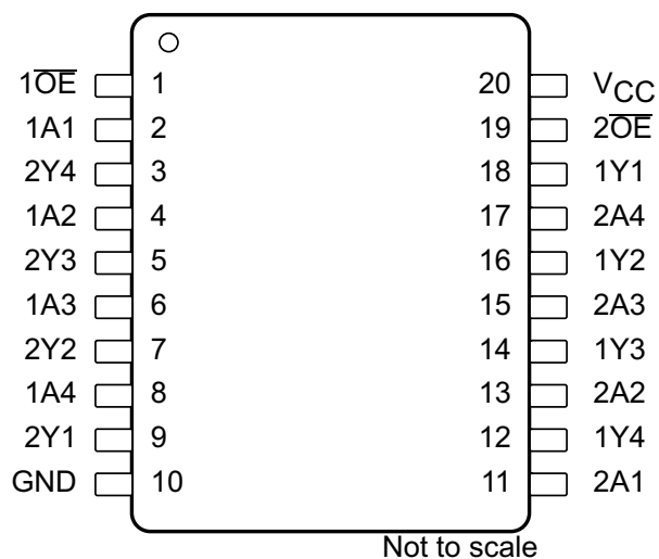
图 4-2. DB、DGV、DW、N、NS 和 PW 封装 20 引脚 SSOP、TVSOP、SOIC、PDIP、SO 和 TSSOP 前视图
