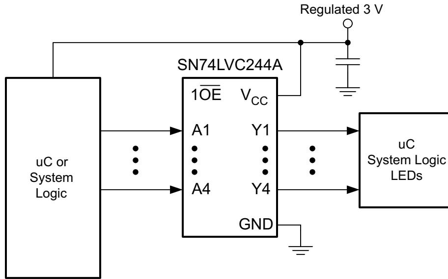
图 8-1. 应用原理图
