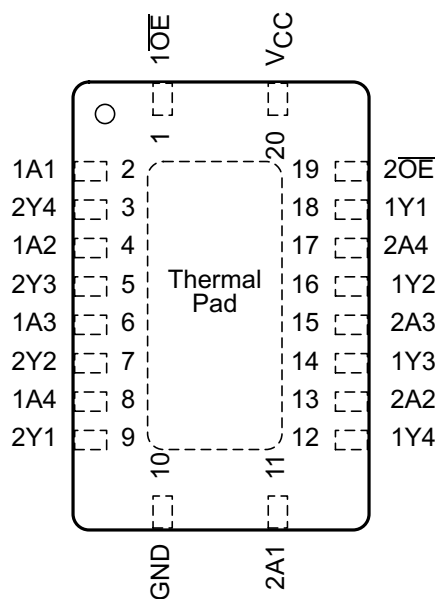
图 4-3. RGY 和 RKS 封装 20 引脚 VQFN 顶视图
